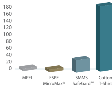
Permeabilidad al aire del tejido - cfm
